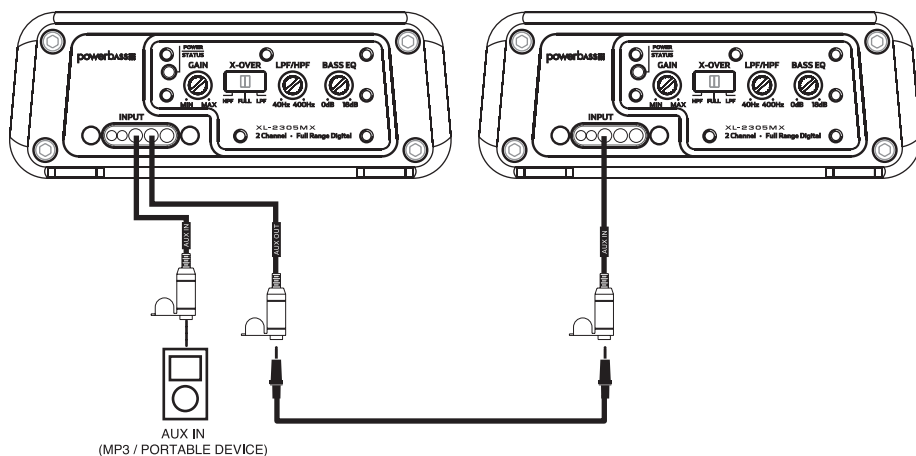
Fig.10 AUX Input using 1/8" (3.5mm)
